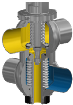
Reinigung: Oberes Ventilgehäuse
