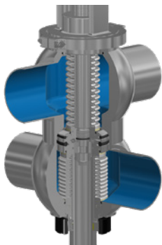
Ventilstellung „OFFEN“
