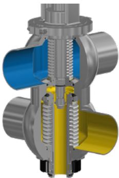
Reinigung: Unteres Ventilgehäuse
