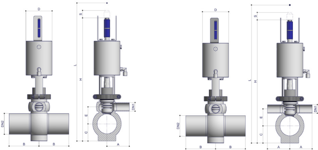
mit Spülstutzen
