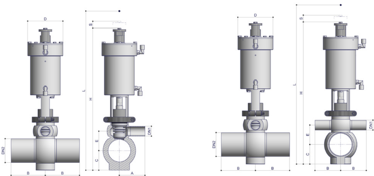
mit Spülstutzen
