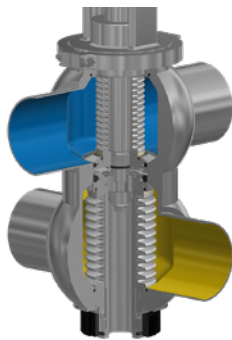
Ventilstellung „ZU“
